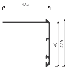
1:2 2080 338 gr/m 6.0m
