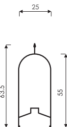
8141 387 gr/m 6.0m
