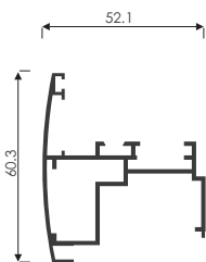
17677 876 gr/m 6.0m
