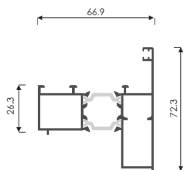
1:3 5211 1.265 gr/m 6.0m
