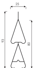
1083 538 gr/m 6.0m
