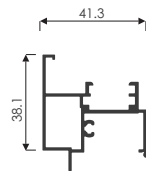
2133 686 gr/m 6.0m
